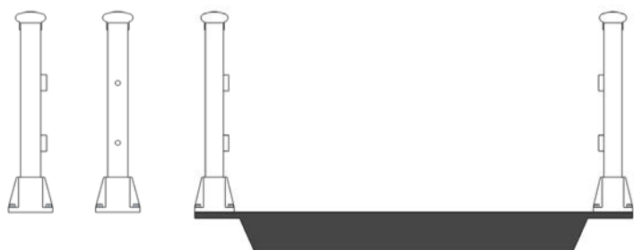
CS® brug - Bevestiging leuning op het dek.
